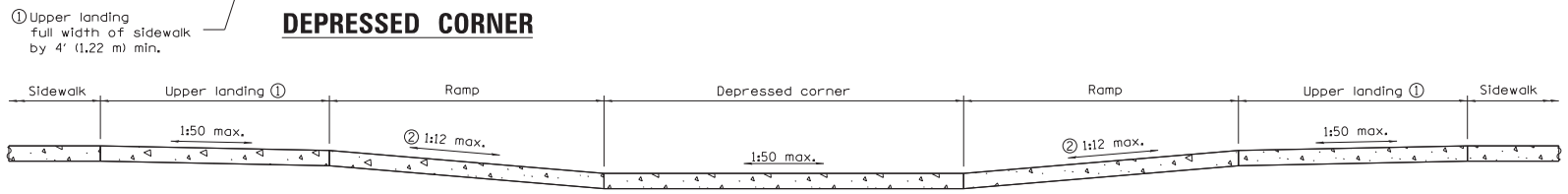
SECTION A-A
